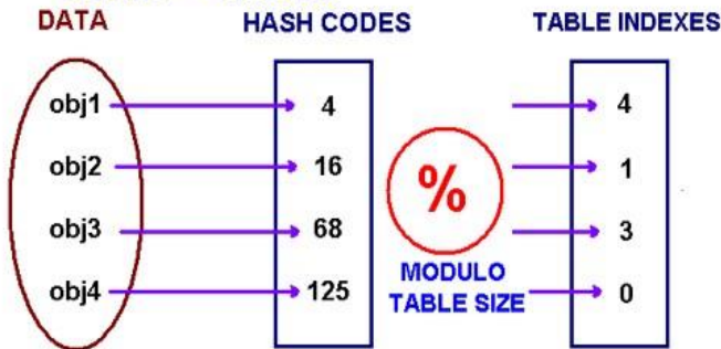
HASH TABLE
